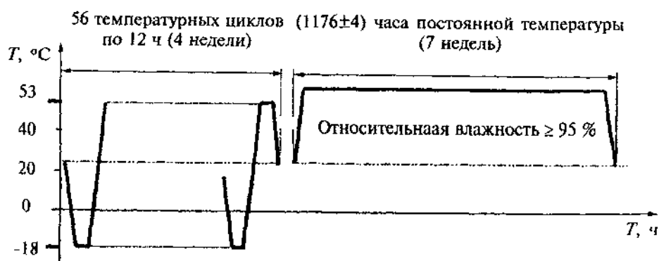
Рис. А.1. График испытаний стеклопакетов по режиму IV
